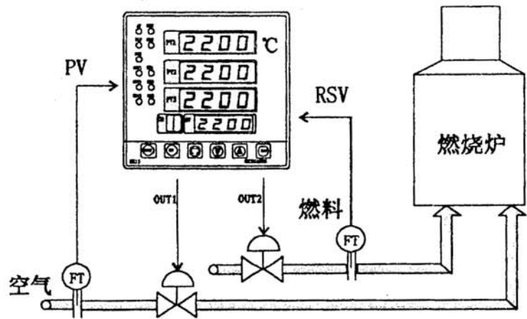
MR13的比值调节
