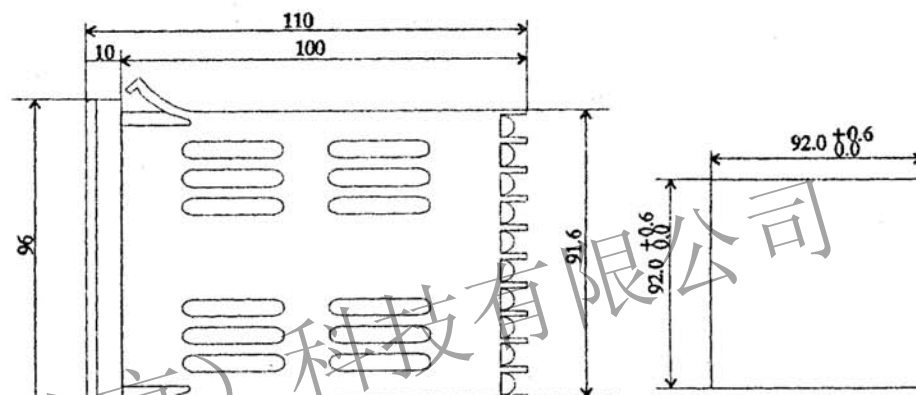
MR13外型及开口尺寸
